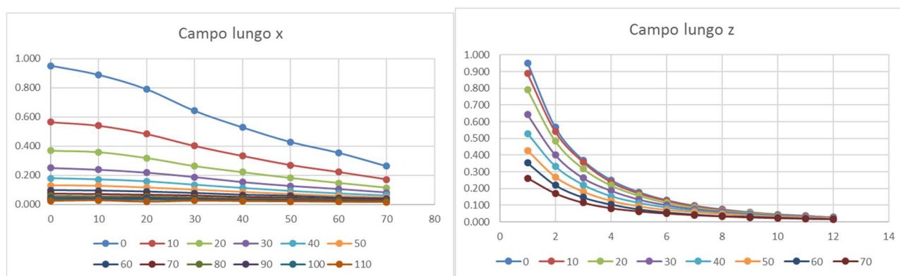
Fig. 3.1 Profili di campo lungo le direzioni x e z, @y=160 cm
