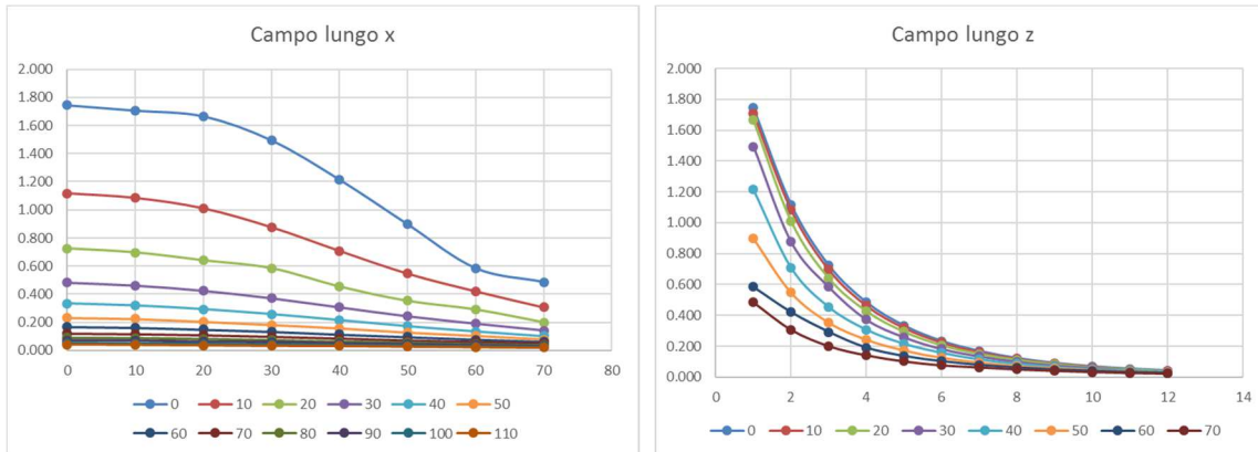
Fig. 2.1 Profili di campo lungo le direzioni x e z, @y=138 cm
