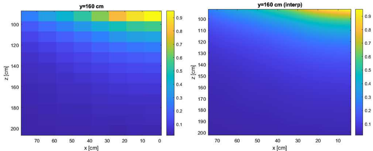
Fig. 3.2 Mappa di campo sul piano xz, @y=160 cm: campo misurato (sinistra), campo interpolato con risoluzione 1x1 cm (destra)
