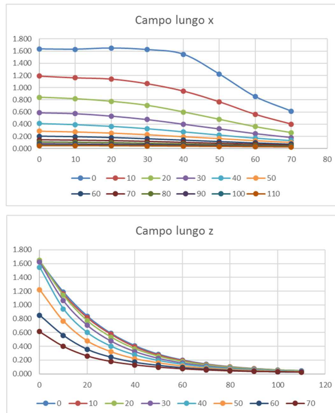
Fig. 1.1 Profili di campo lungo le direzioni x e z, @y=95 cm
