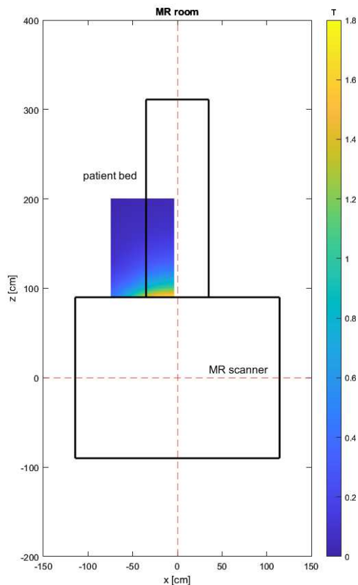
Fig. 1.3 Mappa del campo sul piano xz @y=138 cm localizzata sulla vista dall'alto dello scanner
