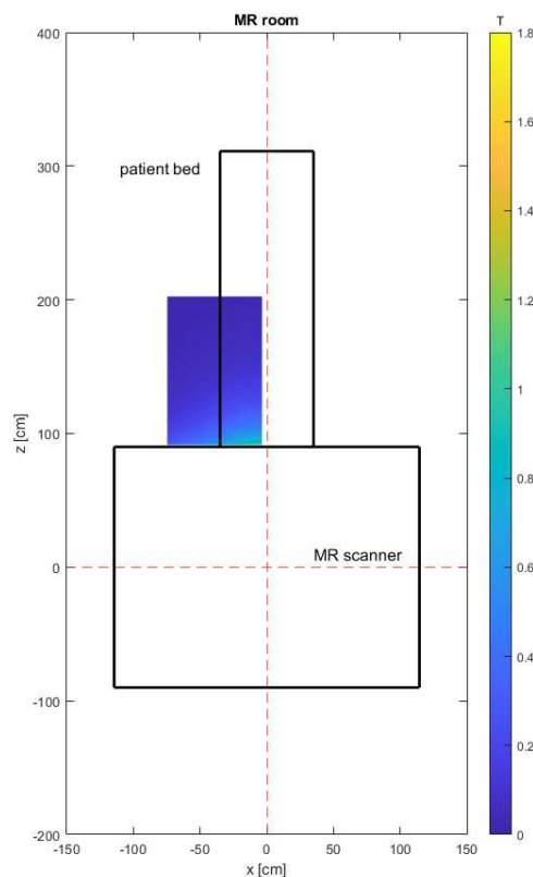
Fig. 3.3 Mappa del campo sul piano xz @y=160 cm localizzata sulla vista dall'alto dello scanner
