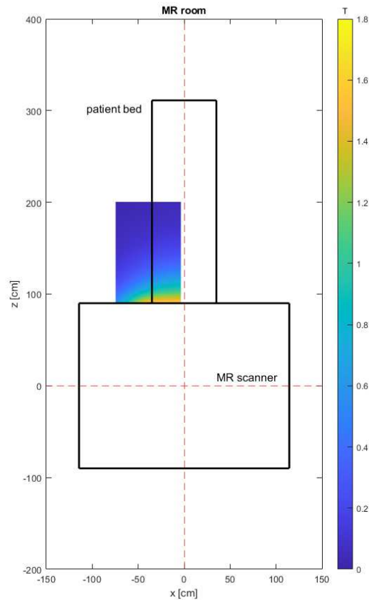
Fig. 1.3 Mappa del campo sul piano xz @y=95 cm localizzata sulla vista dall'alto dello scanner
