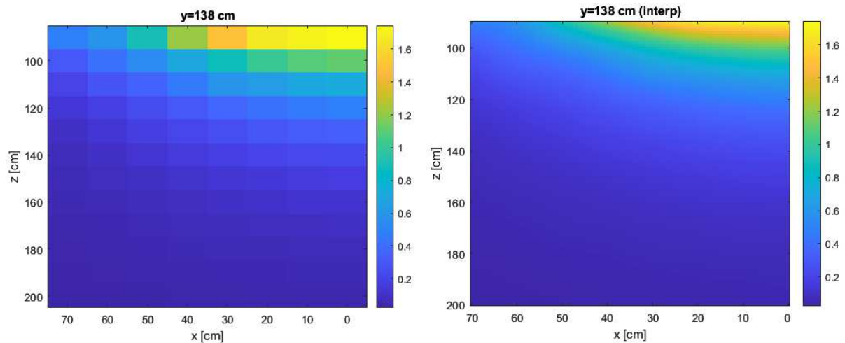
Fig. 2.2 Mappa di campo sul piano xz, @y=138 cm: campo misurato (sinistra), campo interpolato con risoluzione 1x1 cm (destra)
